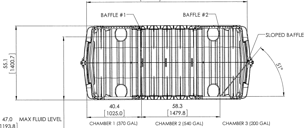
SECTION A-A
